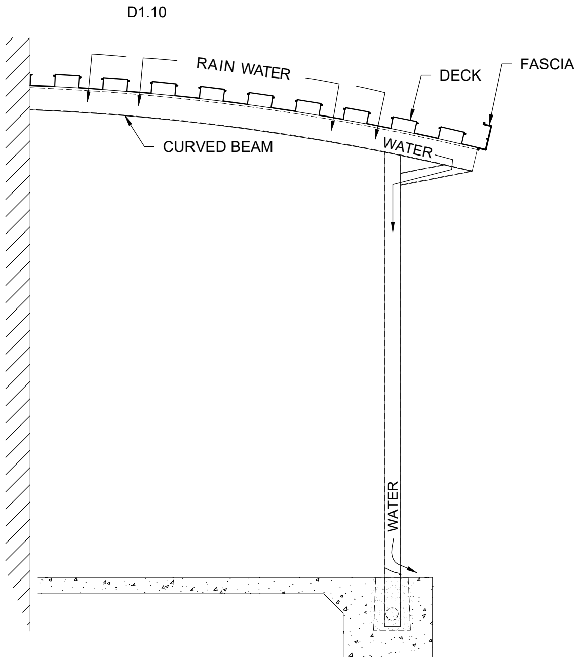
BARREL VAULT L-BENT
