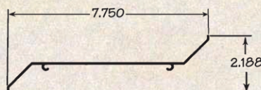
6" Z BLADE
